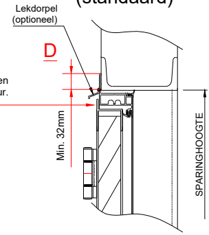
Bovenaansluiting (standaard)
