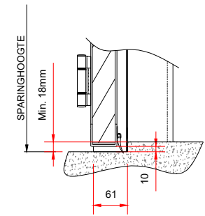
Dorpelaansluiting Optie 2 (excl. dorpel)
