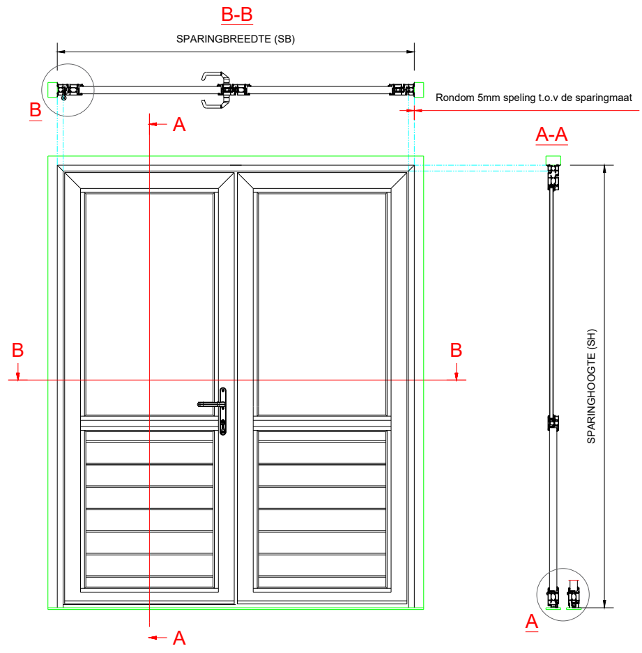
Standaard dorpelaansluiting
