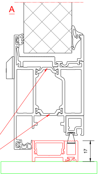
Standaard dorpelaansluiting
