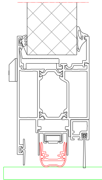
Valdorpel (optioneel)
