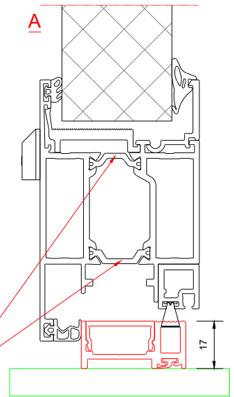
Standaard dorpelaansluiting
